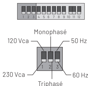
Figure 9 : Commutateurs DIP
