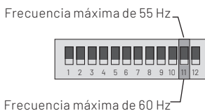
Figura 15: Funcionamiento en frecuencia máxima
