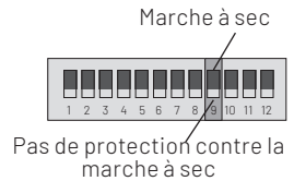
Figure 13: Indicateur de la protection contre la Marche à sec utilisant un commutateur magnétique
