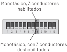
Figura 12: Opción monofásica de 3 conductores
