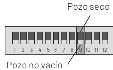
Figura 13: Indicador de pozo seco a través del interruptor magnético
